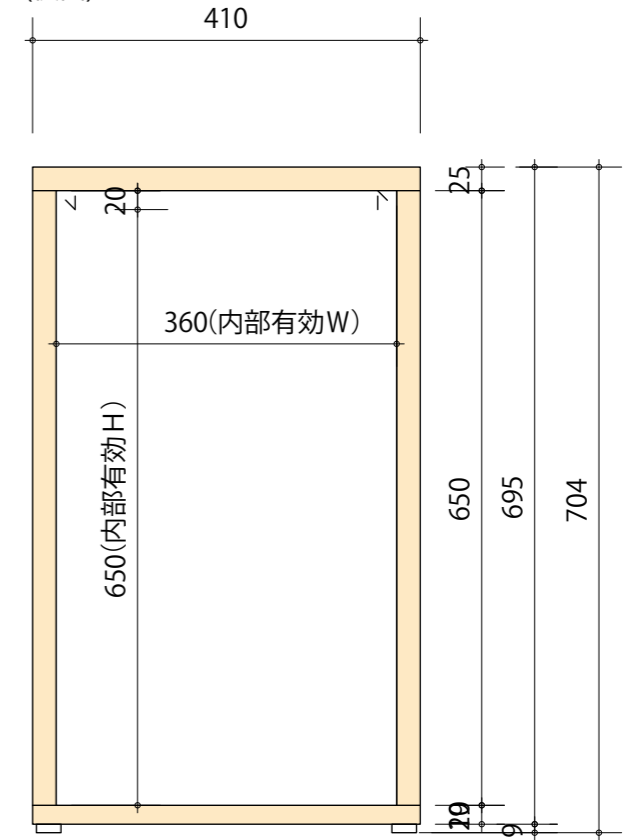
(後面)
