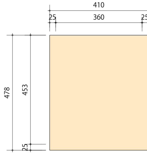
(平面)
