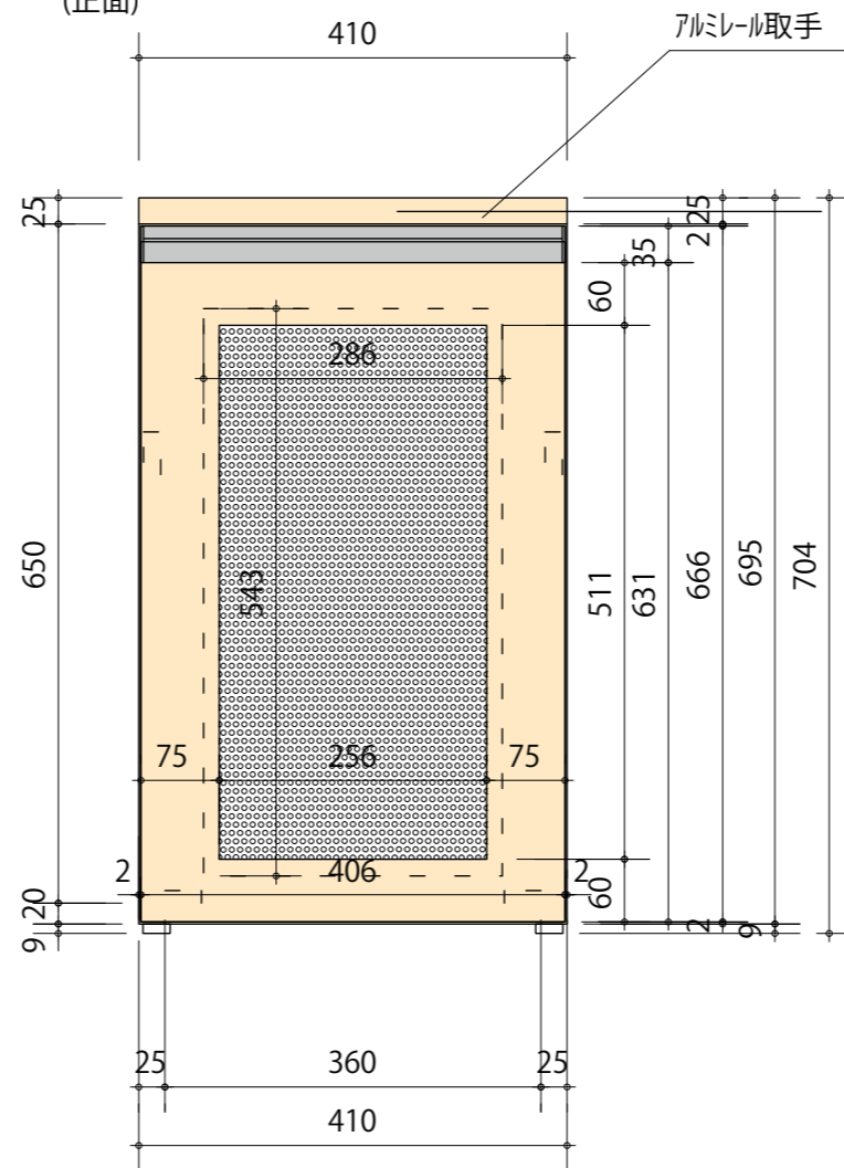
(正面)
