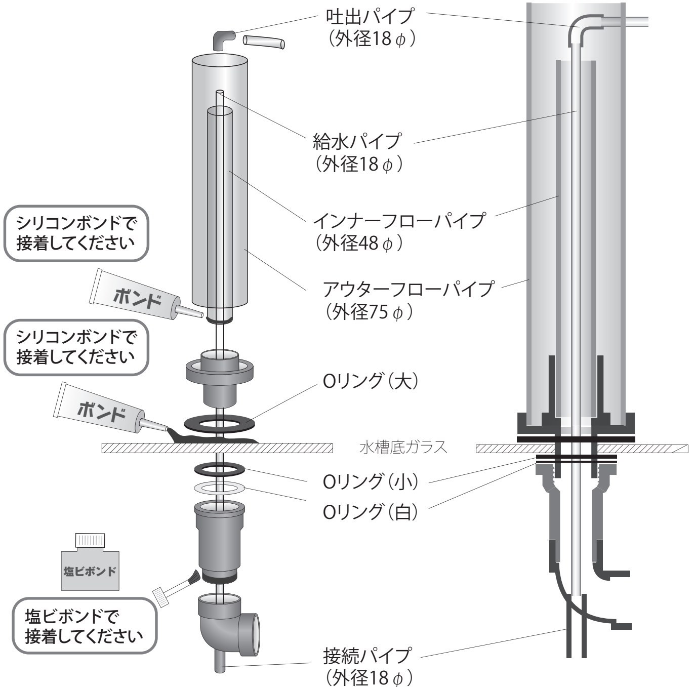
< 配管図 >
